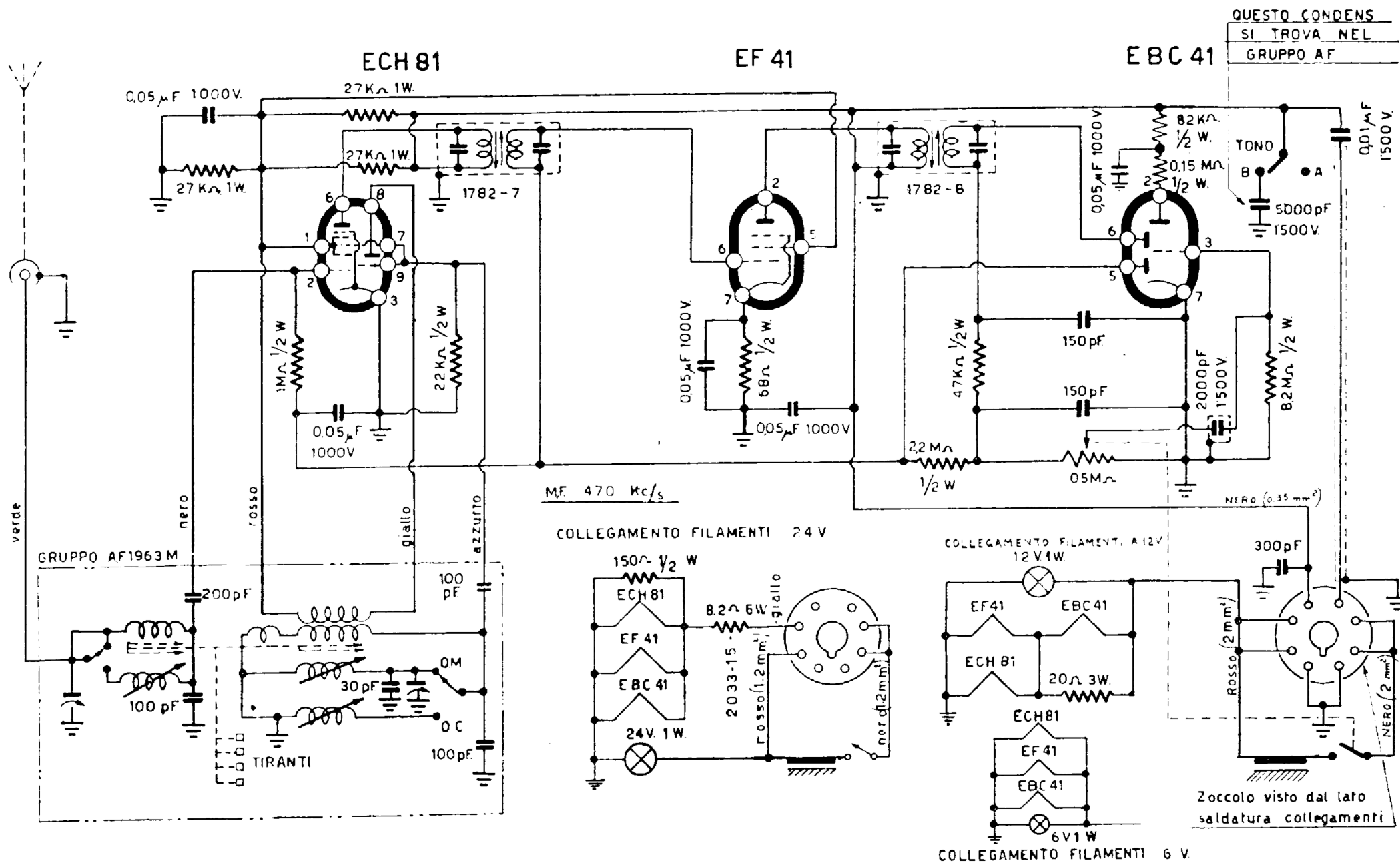
GALLO-CONDOR - Sintonizzatore per autoradio mod. T5 - Due gamme d'onda, medie e corte, con commutazione a tiranti. Media frequenza a 470 kc/s. Lo schema dell'alimentatore e dello stadio finale è riportato a parte.
